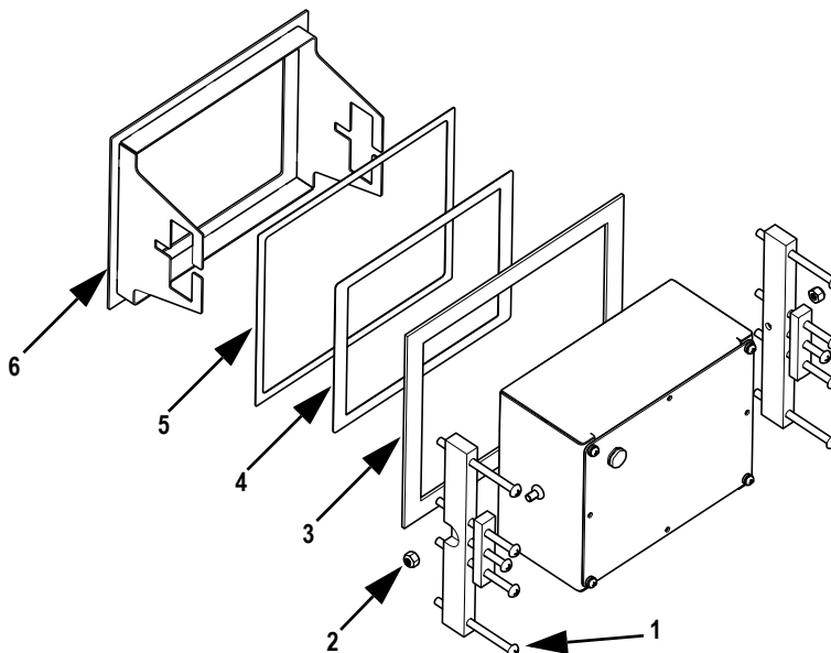
Abbildung 1. Schaltschrankmontagekit
