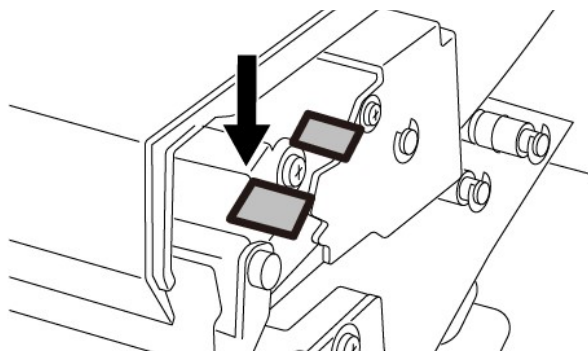
Figura 7-6. Bloquear el cabezal térmico
