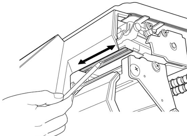
Figura 7-9. Limpiar el cabezal térmico
