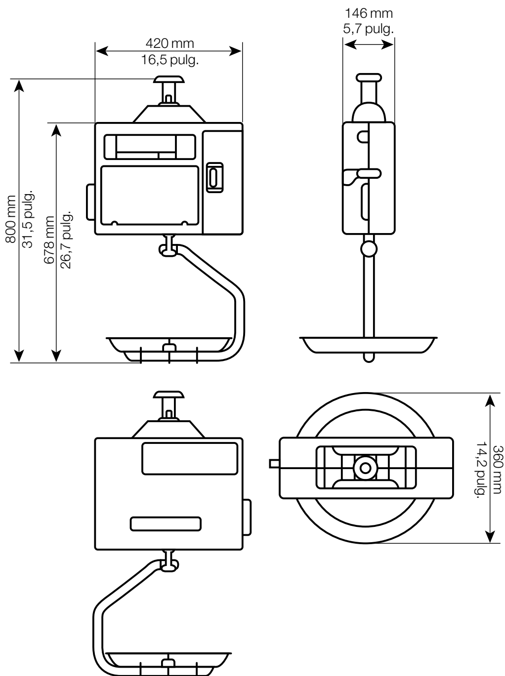
Figura 1-3. Dimensiones exteriores para el Tipo colgante
