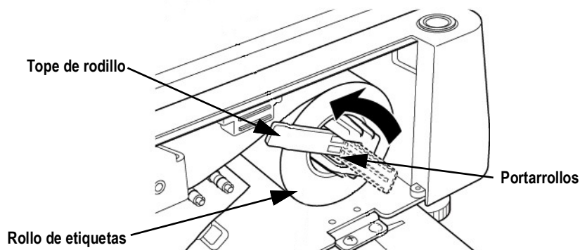
Figura 7-3. Coloque el nuevo rollo en el portarrollos
