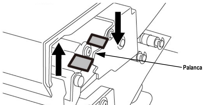
Figura 7-4. Levante la palanca para desbloquear el cabezal térmico
