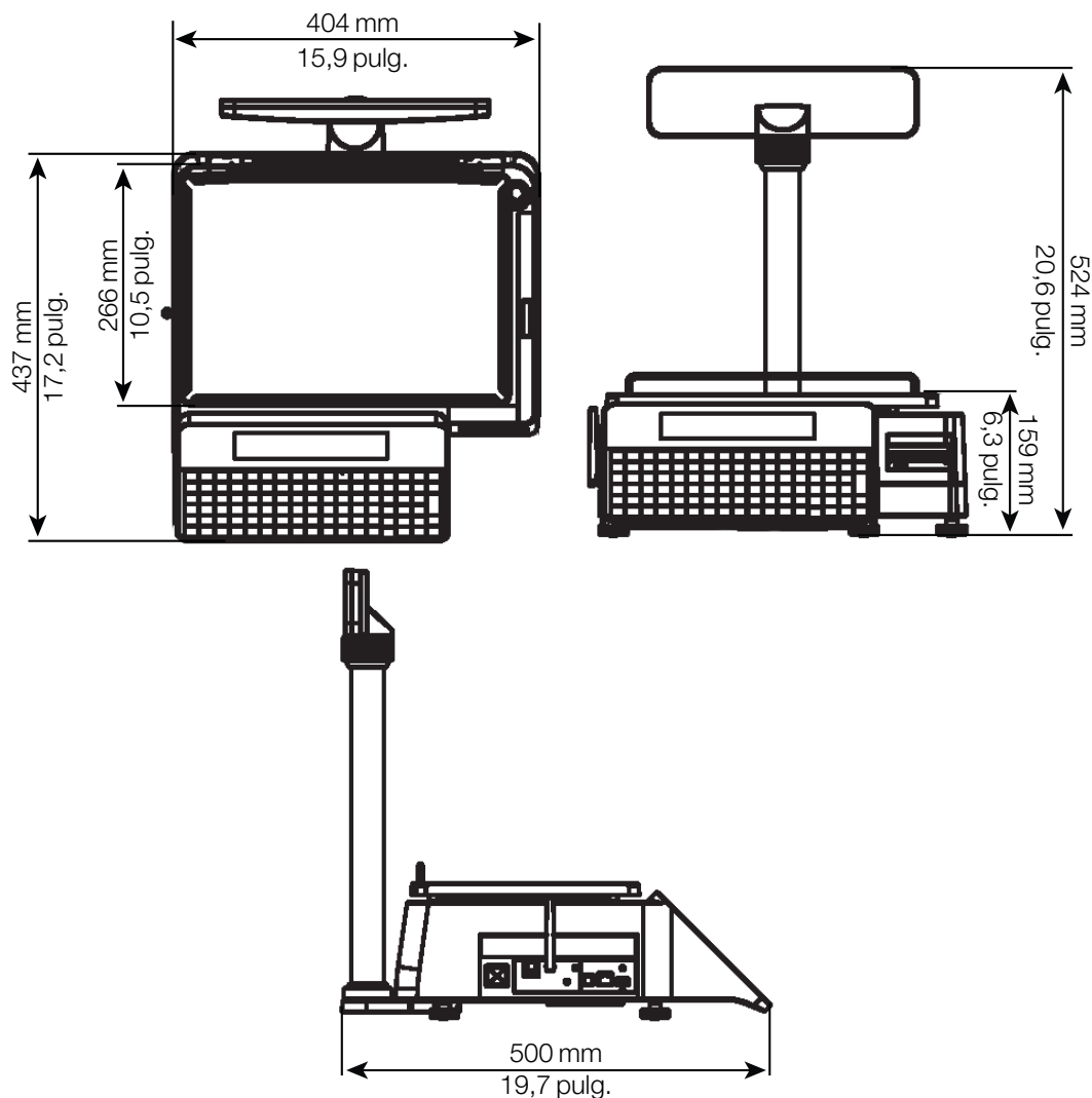
Figura 1-2. Dimensiones exteriores para el Tipo con poste
