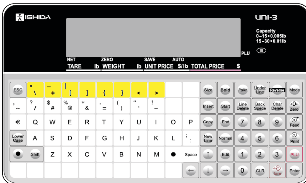
Figura 8-1. Panel de operaciones
