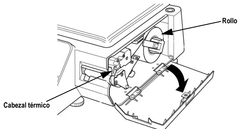
Figura 7-2. Abra la tapa derecha
