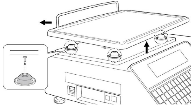
Figura 7-7. Retirar el plato de pesaje
