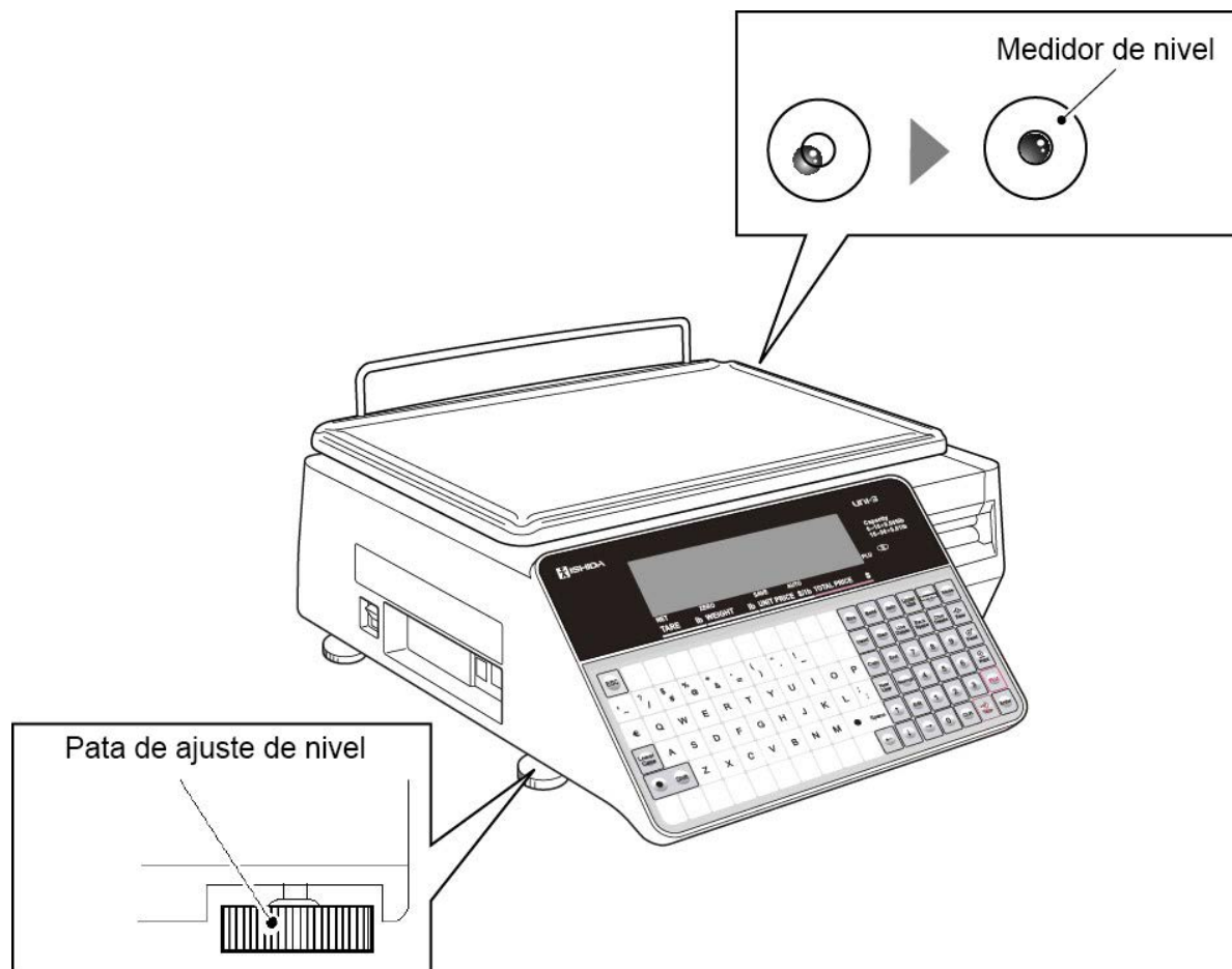
Figura 7-1. Ajuste del nivel
