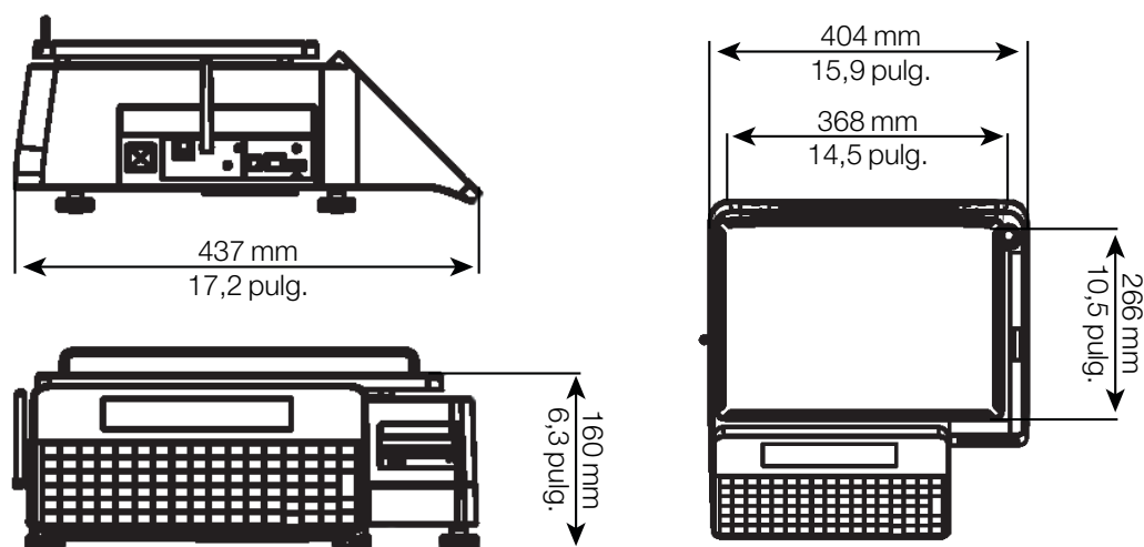
Figura 1-1. Dimensiones exteriores para el Tipo con banco
