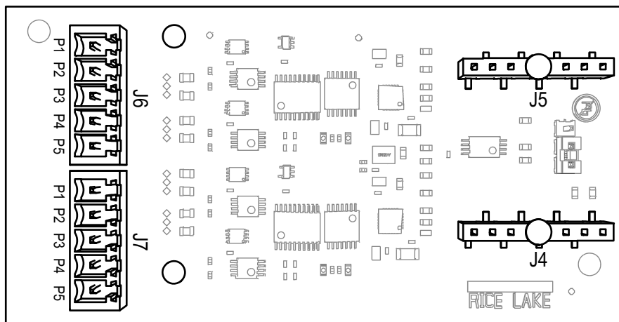
Figura 2. Tarjeta opcional serie doble (vista superior)
