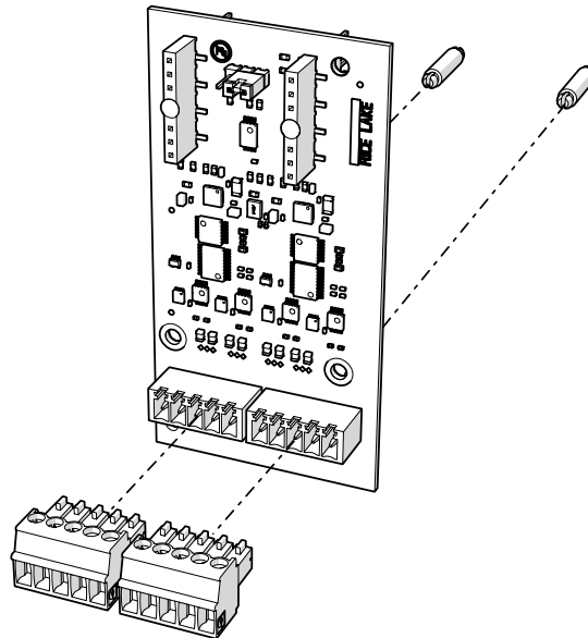
Figura 1. Juego de la tarjeta opcional serie doble
