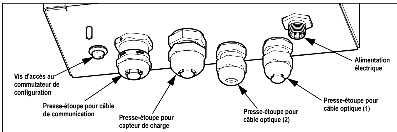
Figure 2-7. Affectation recommandée des presse-étoupes
