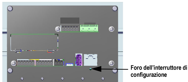
Figura 2-27. Foro dell'interruttore di impostazione e configurazione
