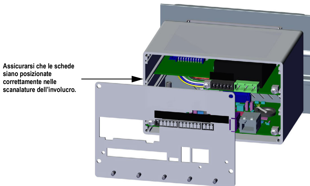
Figura 2-12. Schede installate nell'involucro del gruppo controller
