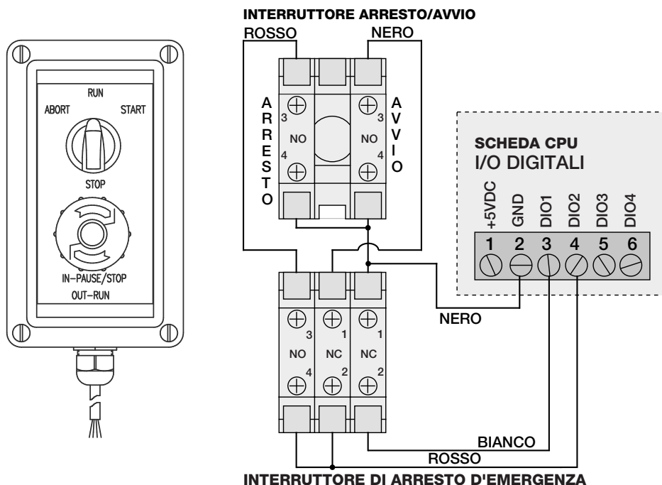
Figura 8-1. Esempio di interruttore di batch e schema di cablaggio
