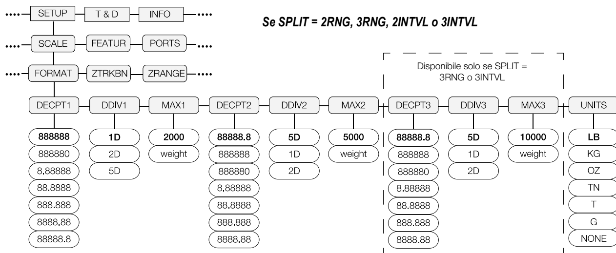
Figura 3-7. Struttura del menu Format con Split 2RNG, 3RNG 2INTVL o 3INTVL
