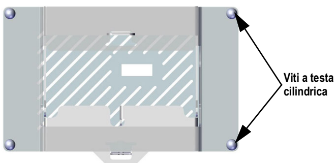
Figura 2-28. Posizioni delle viti della staffa della guida DIN
