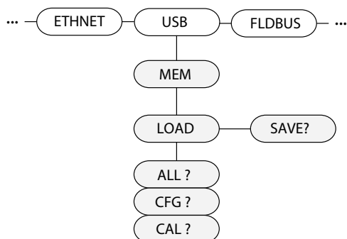
Figura 3-14. Struttura del menu USB Host
