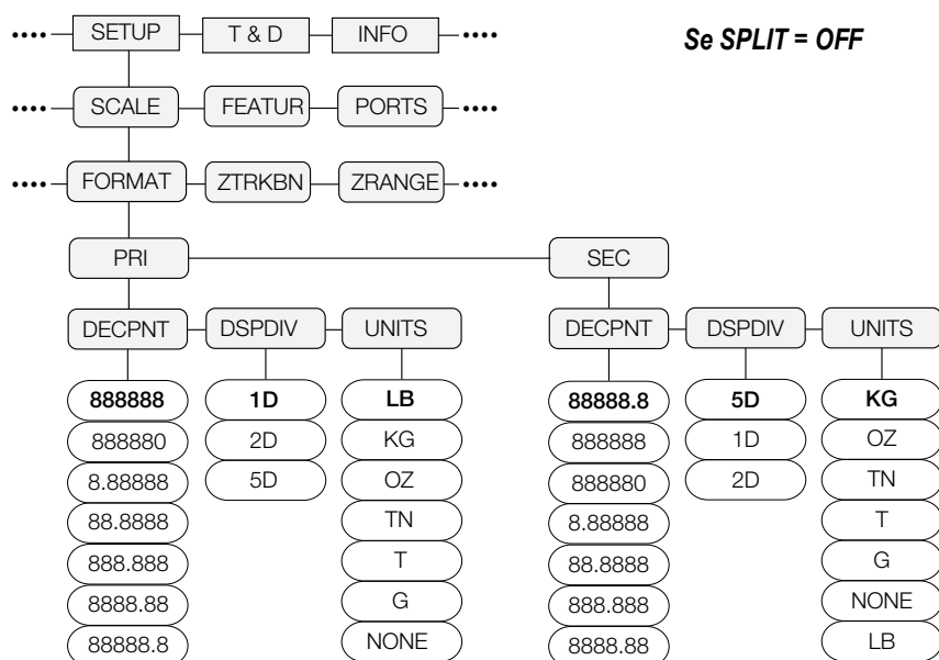
Figura 3-6. Struttura del menu Format con Split Off
