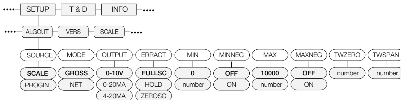
Figura 3-23. Menu Analog Output
