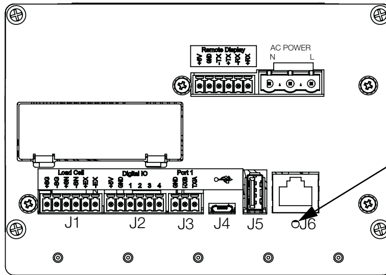
Figura 3-1. Vista posteriore – Accesso all'interruttore di configurazione
