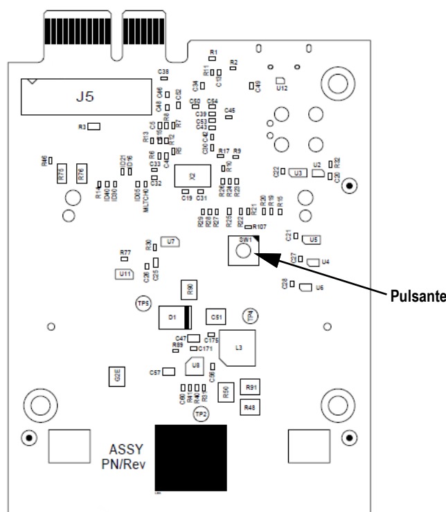
Figura 10-4. Posizione del pulsante sulla scheda host Anybus (PN 164756)
