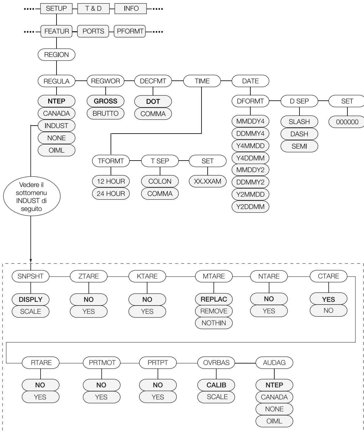
Figura 3-10. Struttura del menu Region
