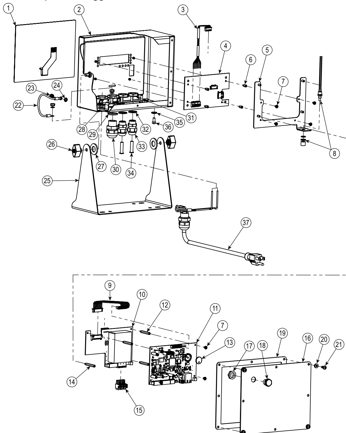
Figura 2-32. Parti per montaggio universale - Illustrazione
