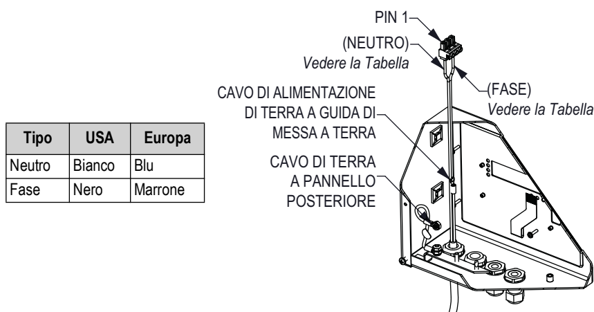
Figura 2-19. Collegamenti di messa a terra
