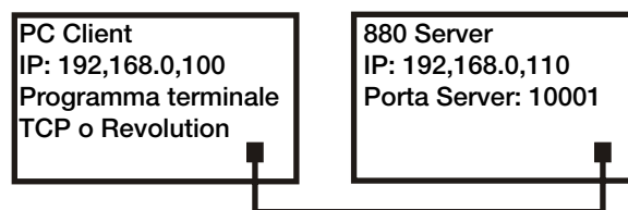
Figura 9-1. Connessione diretta da computer a Ethernet dell'880
