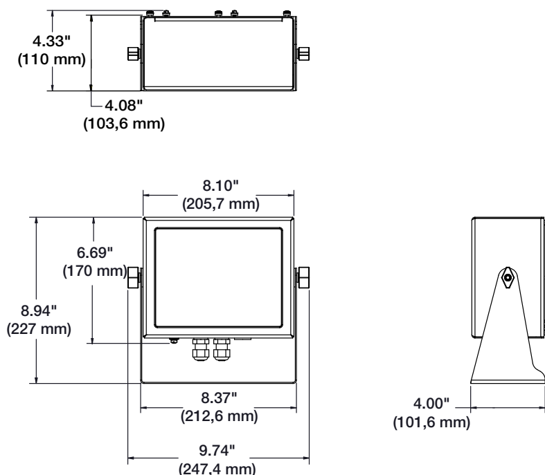
Figura 2-13. Dimensioni del supporto universale
