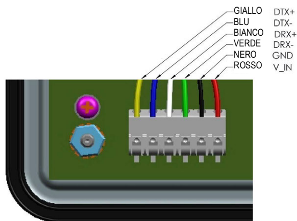
Figura 2-8. Dettaglio del collegamento del fascio di cavi
