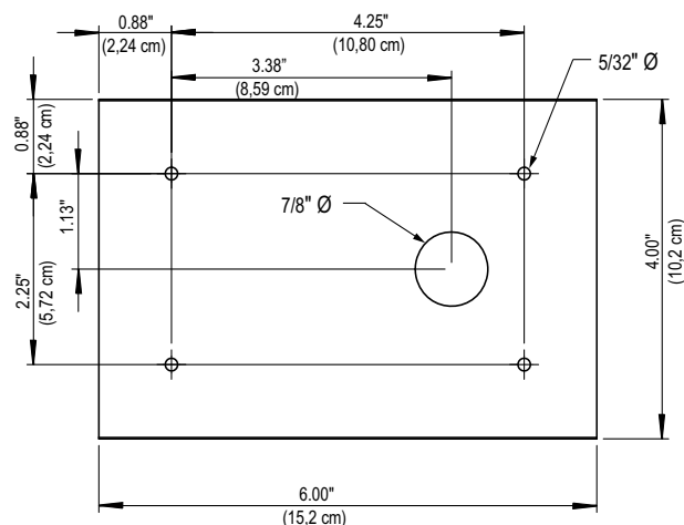
Figura 2-2. Schema per l'esecuzione dei fori
