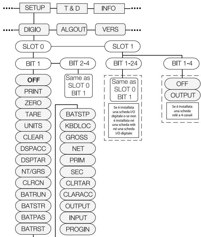
Figura 3-22. Menu Digital I/O
