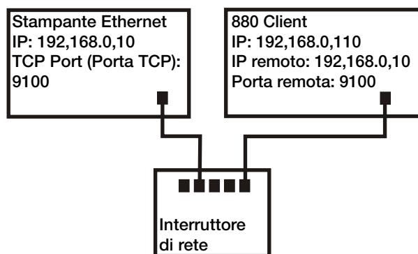
Figura 9-3. Connessione a un host remoto
