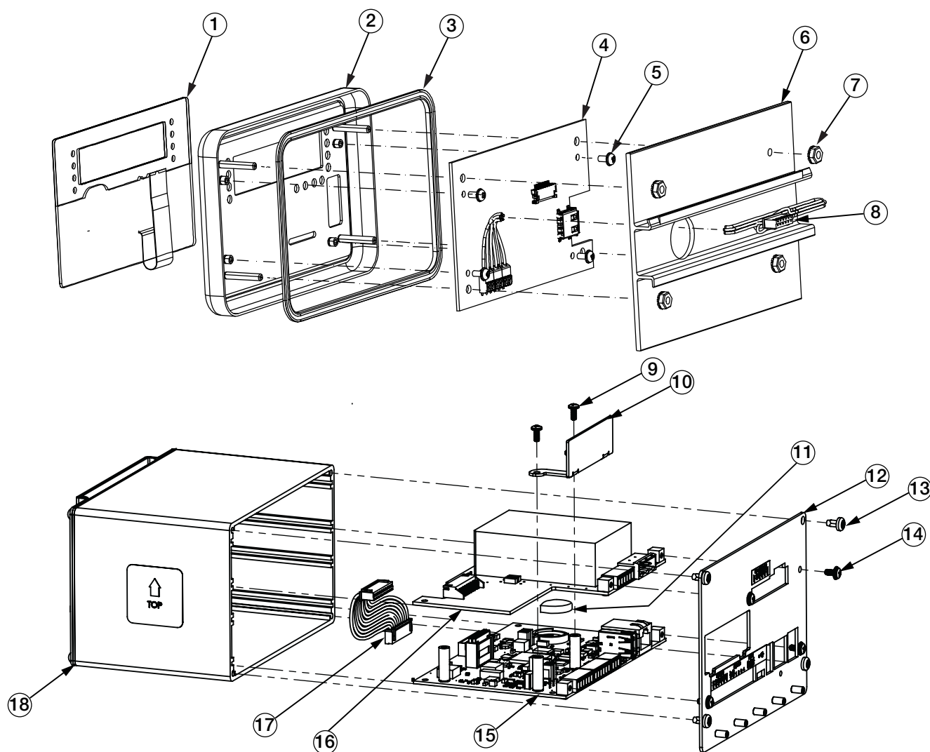
Figura 2-31. Parti per il montaggio a pannello - Illustrazione
