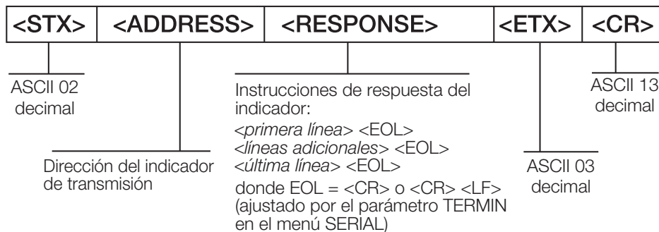
Figura 12-3. Formato de datos de respuesta RS-485
