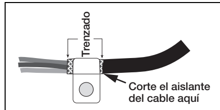
Figura 2-5. Cable con blindaje trenzado
