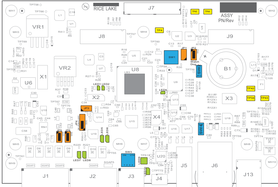
Figura 12-4. Tarjeta del CPU
