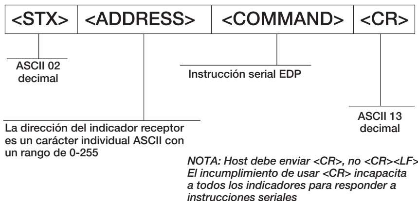
Figura 12-2. Formato de datos de envío RS-485
