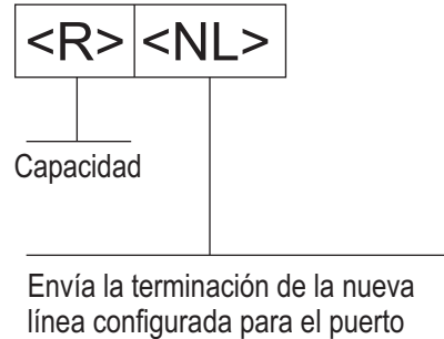
Figura 12-1. Secuencia de formato de datos serial
