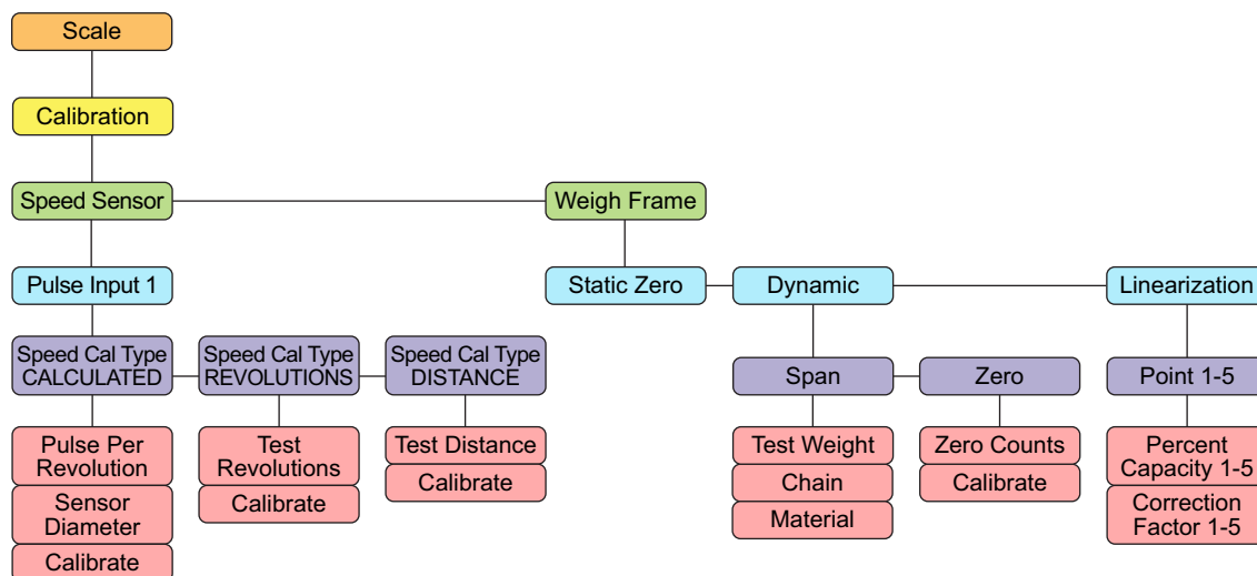
Figura 4-7. Menú Scale – Calibration
