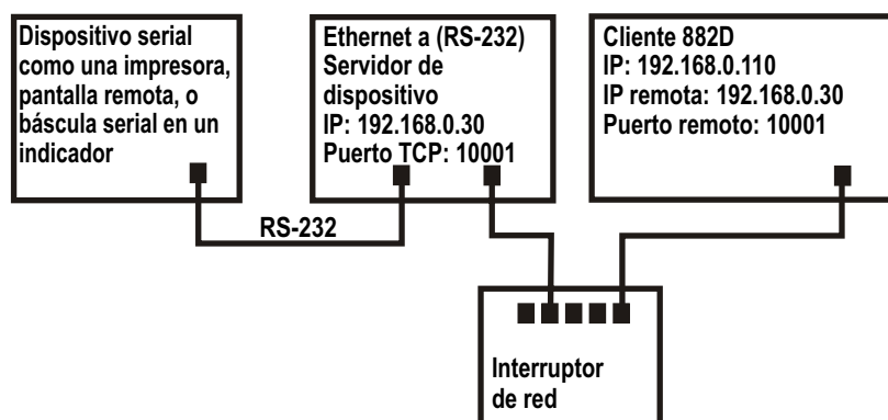
Figura 9-5. Transmita o demande datos a un servidor de dispositivo RS232 de Ethernet remoto
