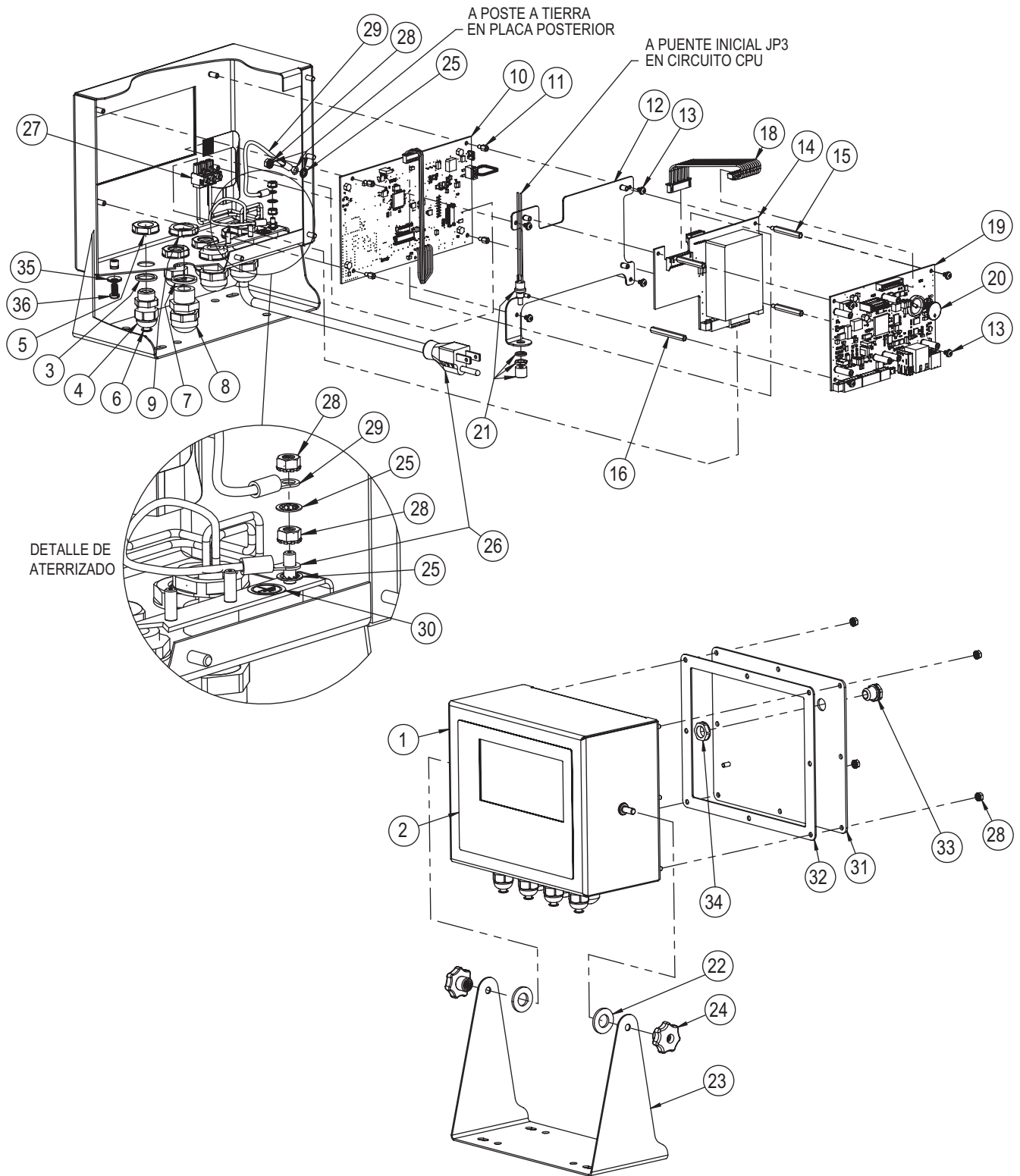
Figura 2-12. Vista ampliada de repuestos
