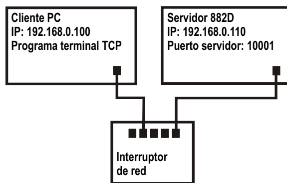
Figura 9-2. Conexión de la PC al Ethernet del 882D a través de un interruptor o router de red
