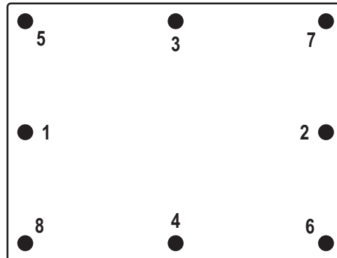
Figura 2-10. Secuencia de apriete
