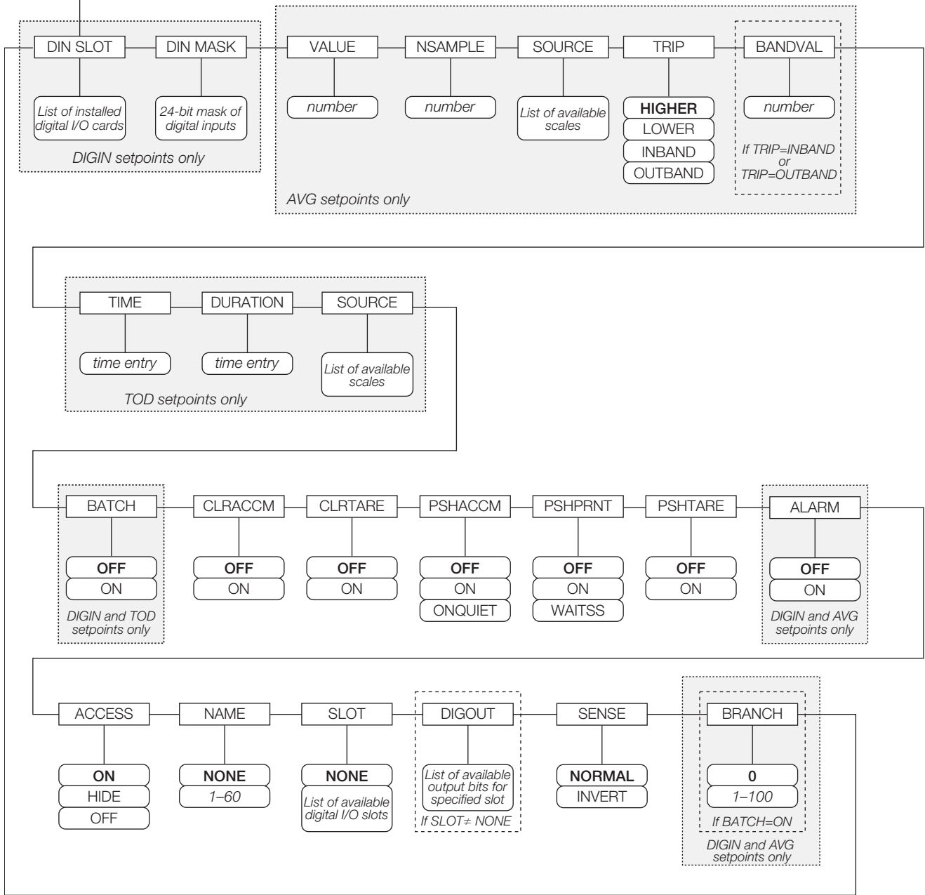
Figura 9-6. Parámetros de Setpoints DIGIN, AVG, y TOD
