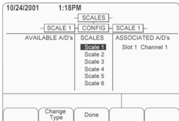
Figura 3-2. Pantalla de Configuración de Báscula
