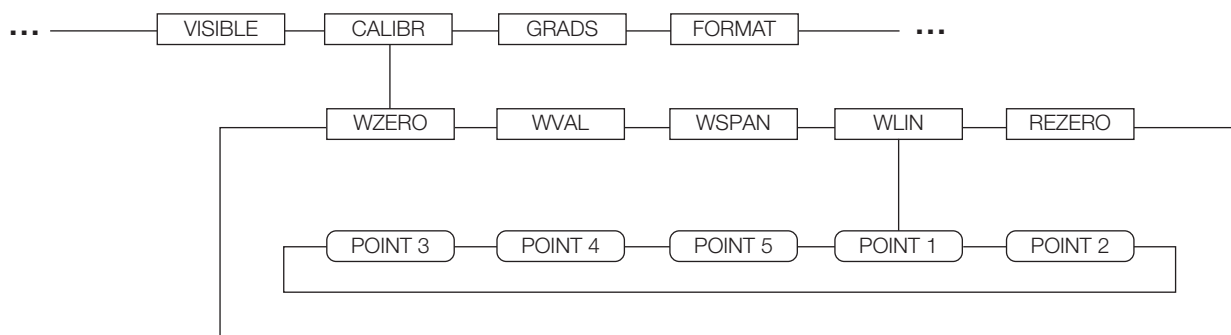
Figura 3-7. Menú SCALES, Submenú CALIBR
