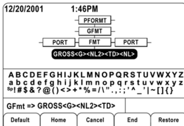
Figura 7-3. Pantalla de Selección de Caracteres en Formateo de Impresión
