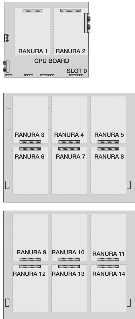
Figura 2-13. Circuito CPU con 2 Circuitos de Expansión de 6 Tarjetas.
