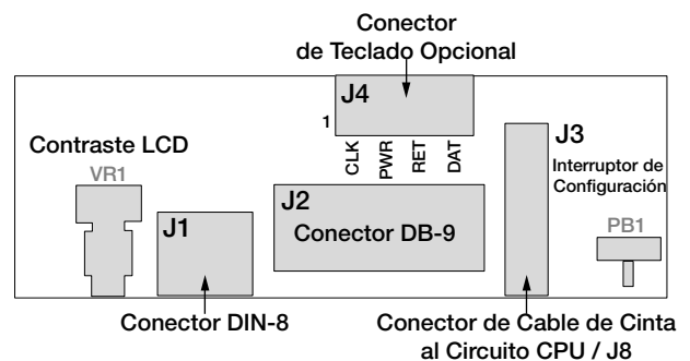
Figura 2-5. Vista Superior del Circuito de Interfaz
