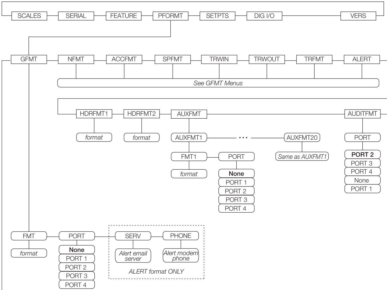
Figura 7-2. Menú PFORMT
