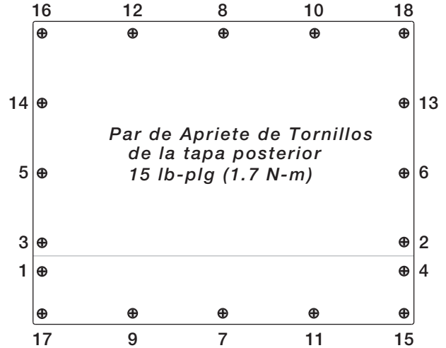
Figura 2-15. Tapa Posterior del Gabinete del 920i
