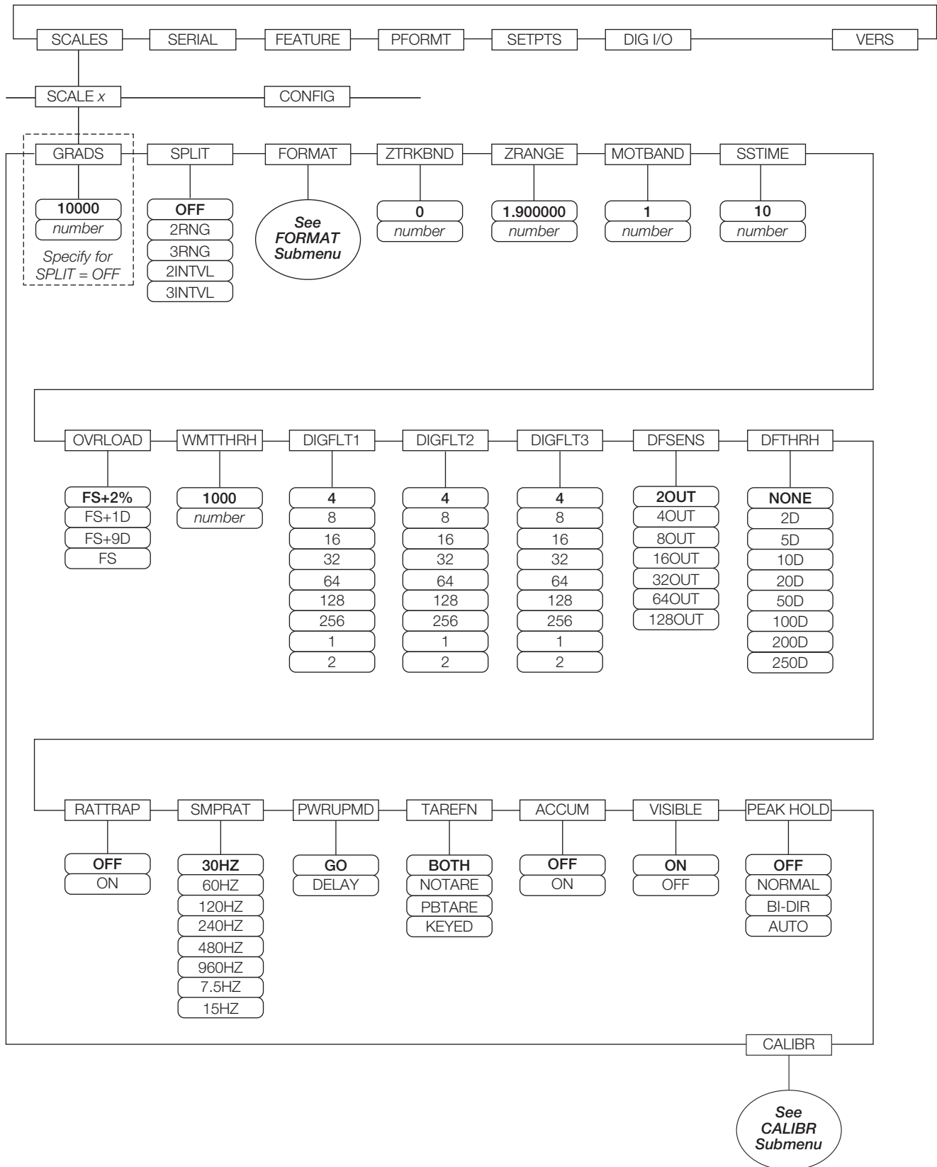
Figura 3-4. Menú SCALES
