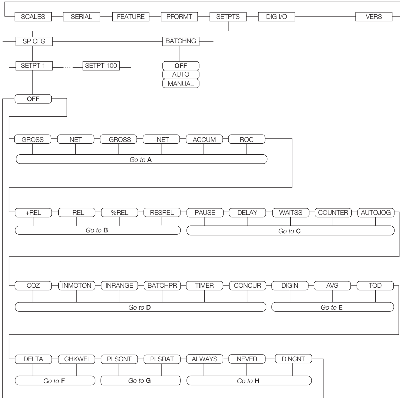
Figura 9-1. Menú SETPTS
