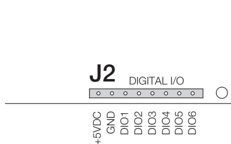
Figura 2-8. Clavijas J2 del Circuito 920i CPU. Revisión H
