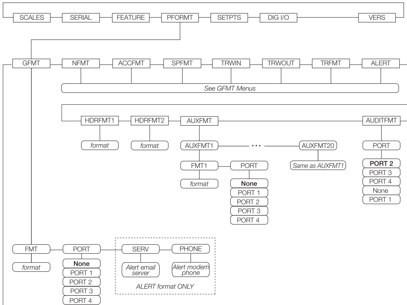
Figura 3-16. Menú PFORMAT
