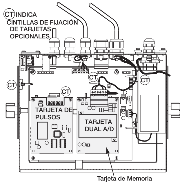
Figura 2-10. Tarjetas Opcionales Instaladas, Mostrando los Cables Asegurados
