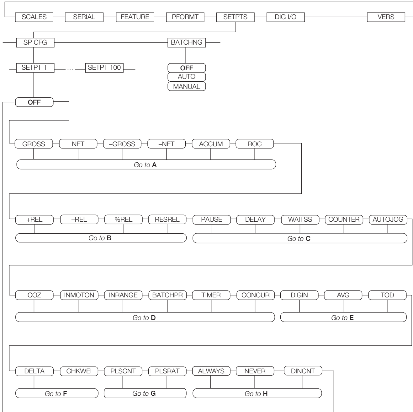
Figura 3-17. Menú SETPTS
