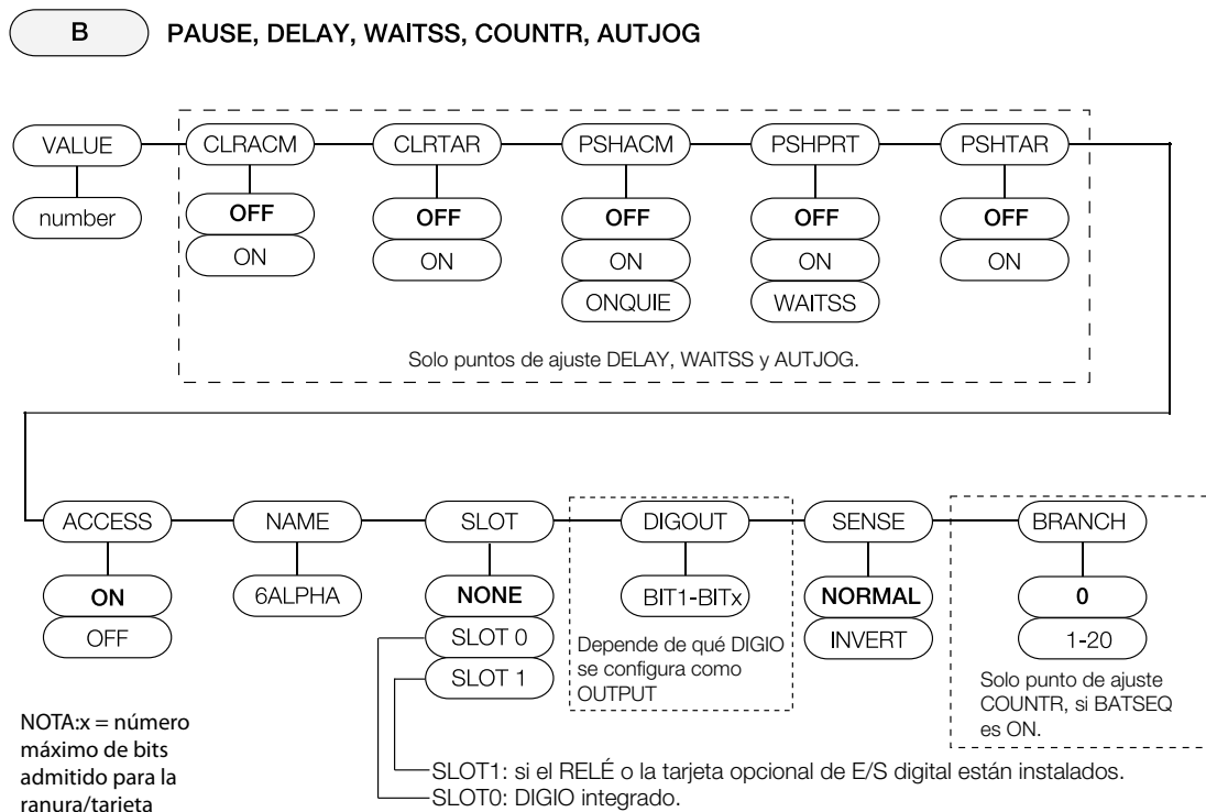
Figura 3-19. Estructura del menú Setpoint - Estructura B
