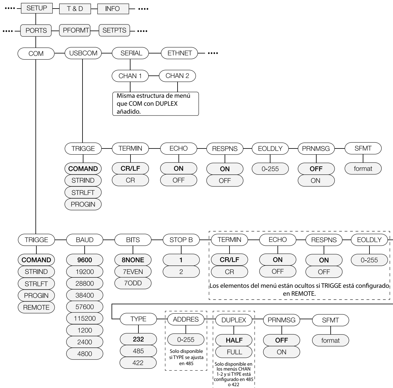
Figura 3-12. Estructura de menús COM, USBCOM y SERIAL
